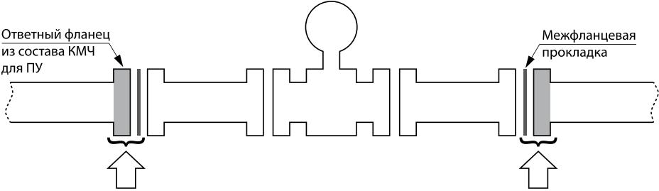
Стрелками показано место установки комплекта КМЧ для переходного участка
