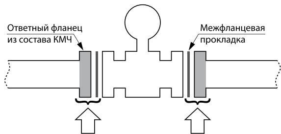
Стрелками показано место установки комплекта КМЧ для расходомера
